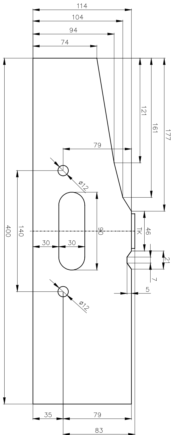
Obr. 2: Výkres mechanického rozhraní tvaru RN
