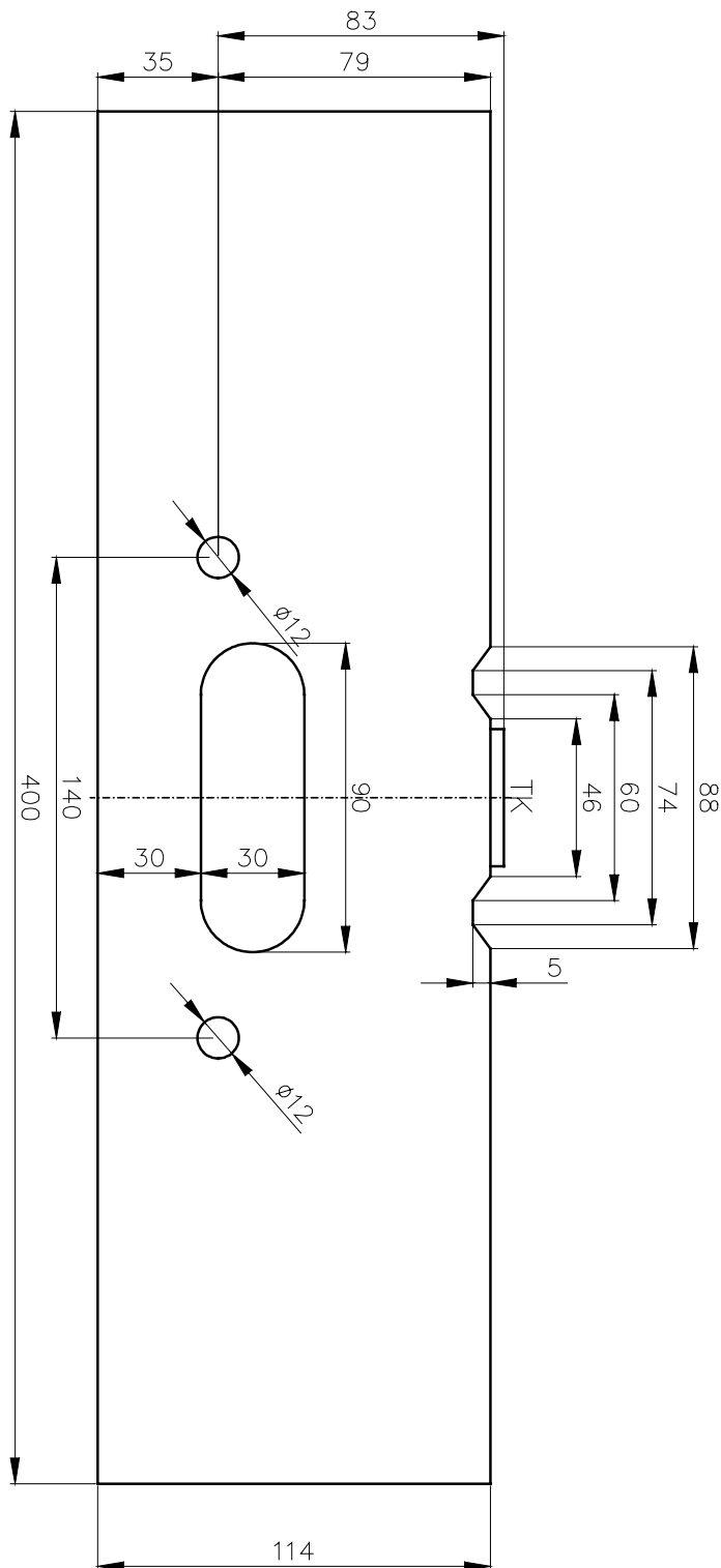
Obr. 1: Výkres mechanického rozhraní tvaru RR
