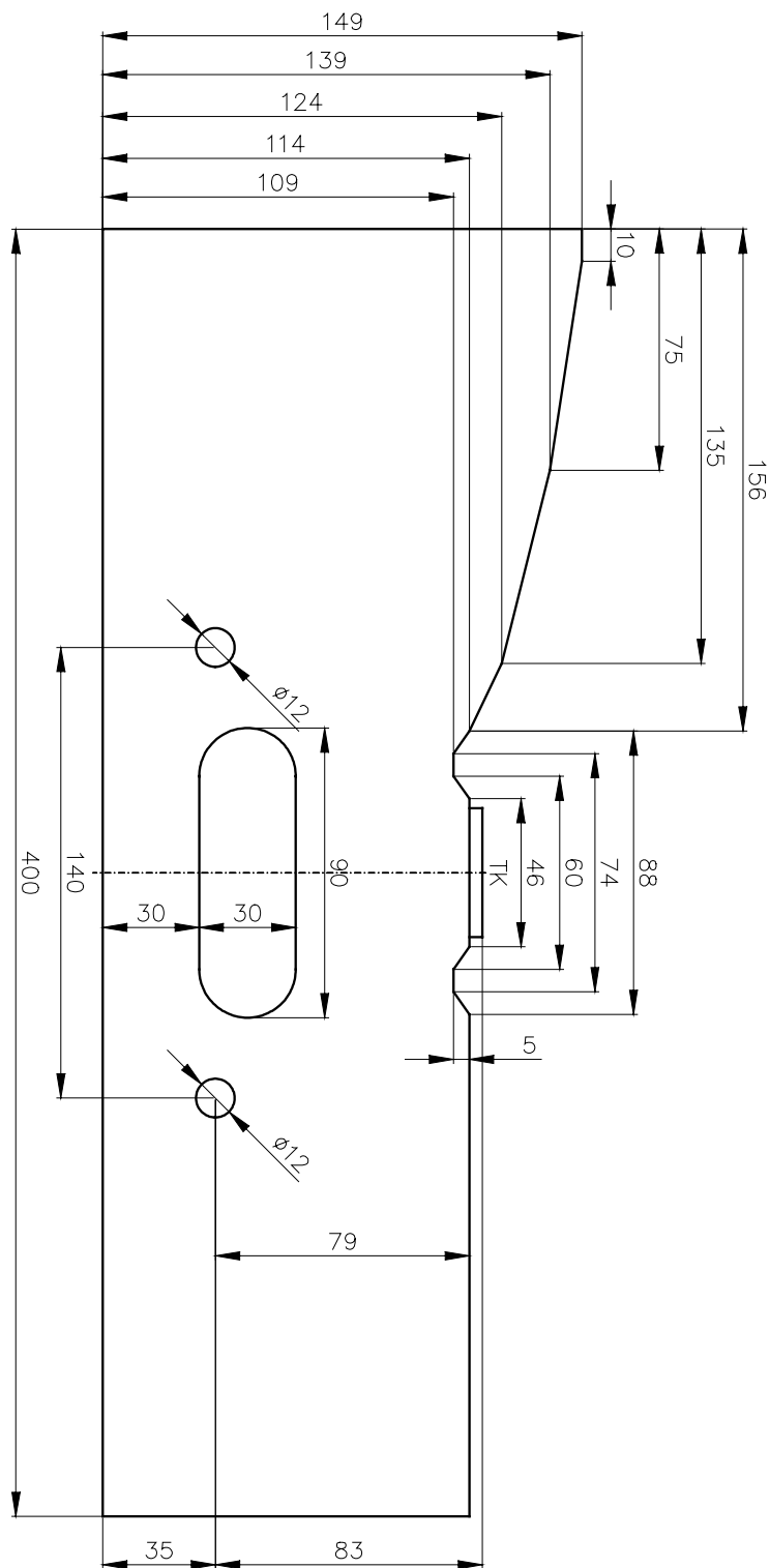
Obr. 4: Výkres mechanického rozhraní tvaru ZR
