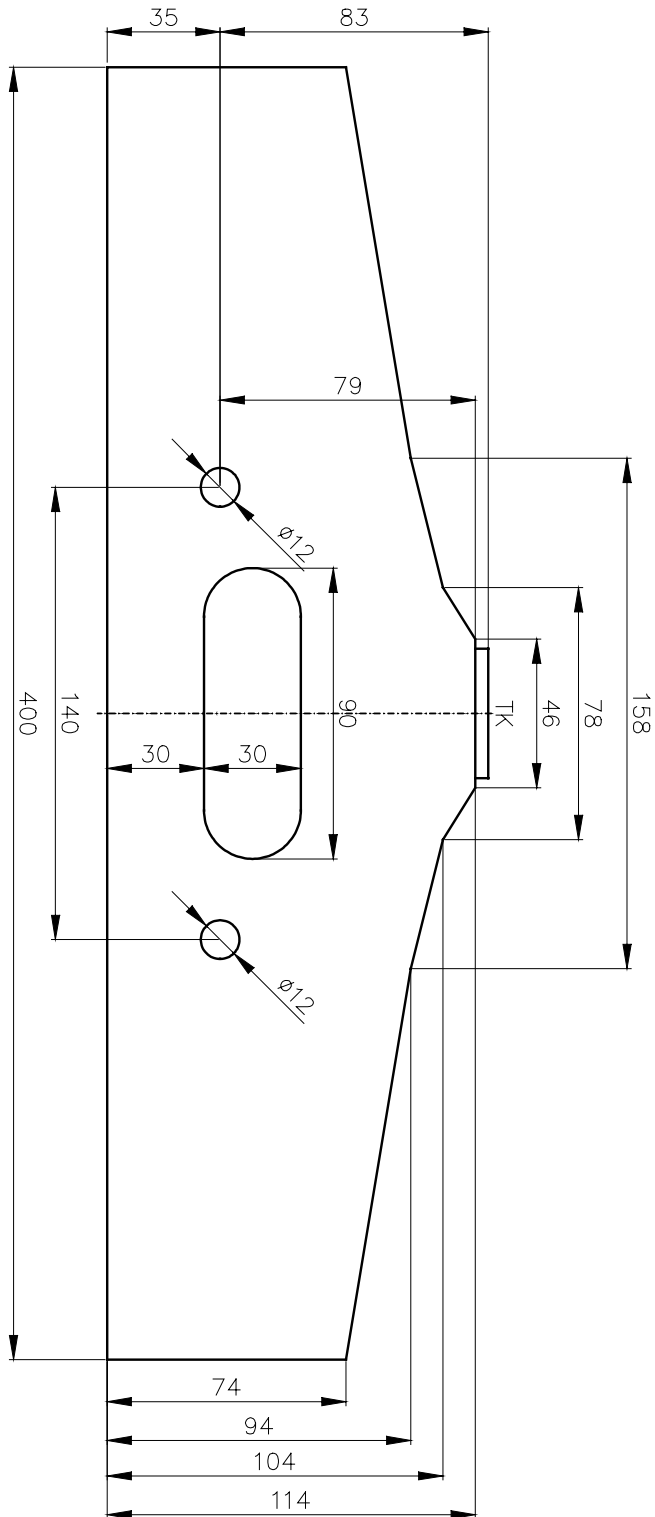
Obr. 3: Výkres mechanického rozhraní tvaru NN
