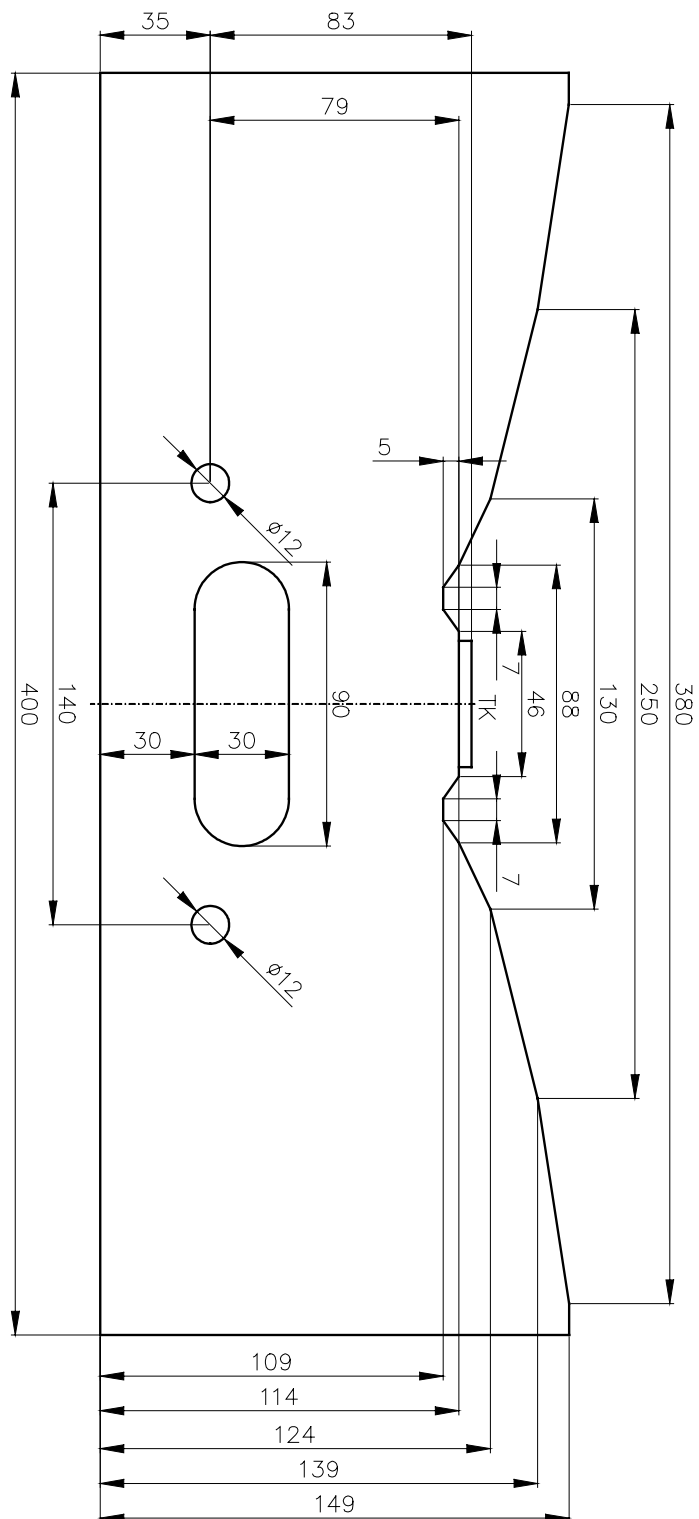
Obr. 6: Výkres mechanického rozhraní tvaru ZZ
