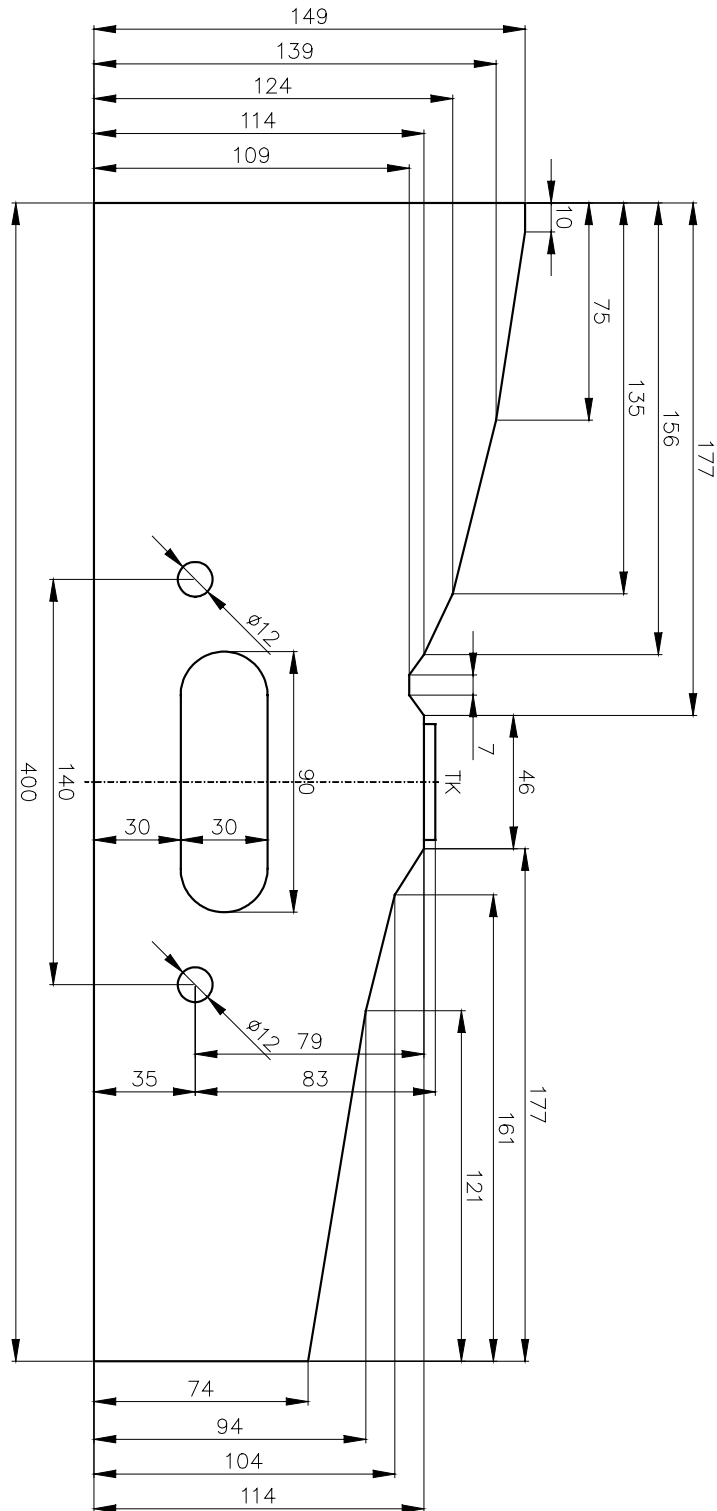
Obr. 5: Výkres mechanického rozhraní tvaru ZN
